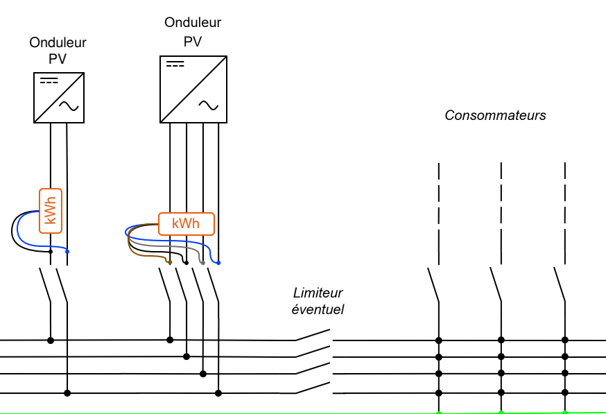
Détail de câblage des compteurs 3P
