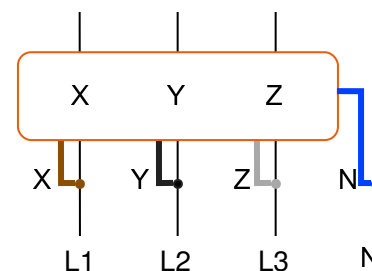
Détail de câblage des compteurs 3P
